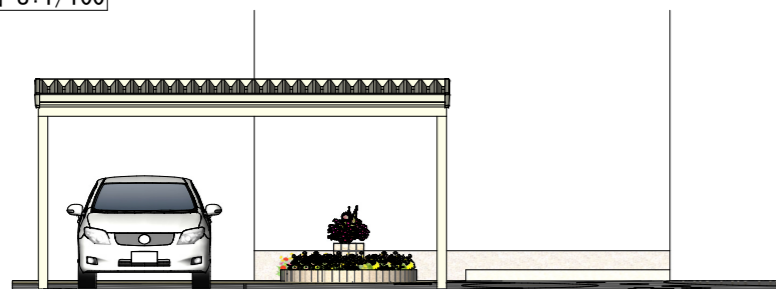
立面図 S:1/100
